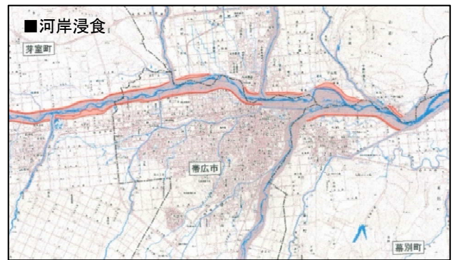
図 2-8 洪水浸水想定区域図 (家屋倒壊等氾濫想定区域 (河岸浸食))
